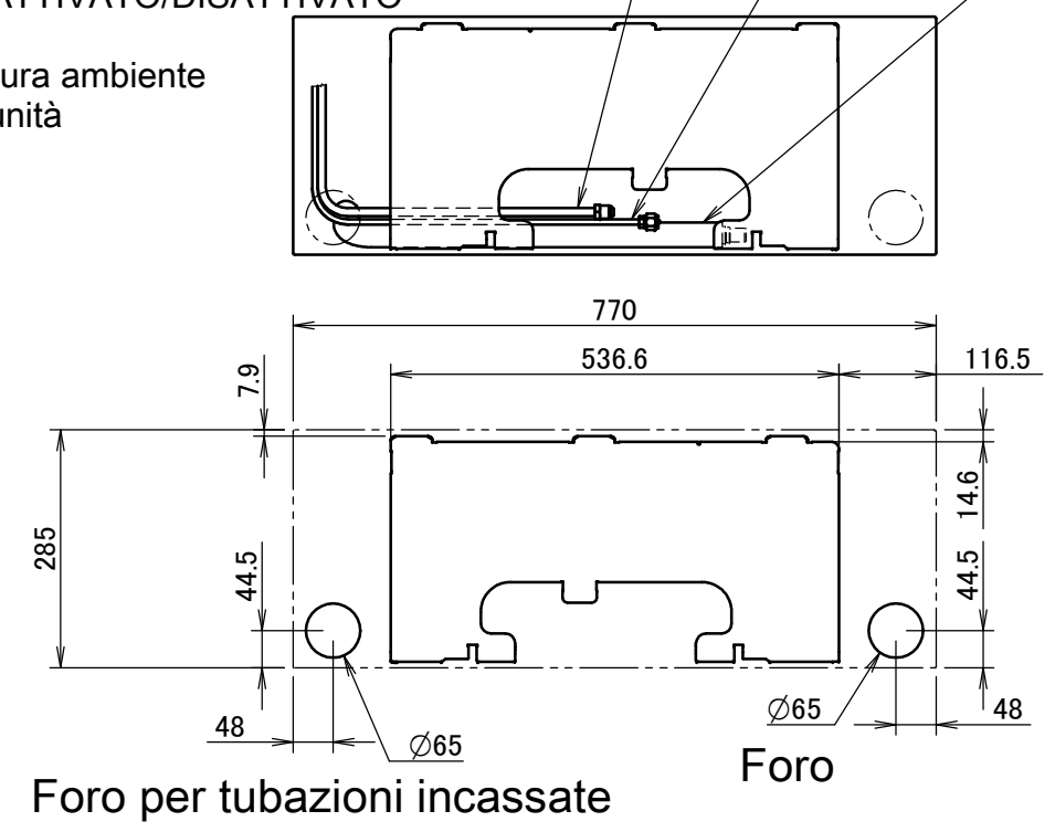
Posizione standard dei fori sulla parete
